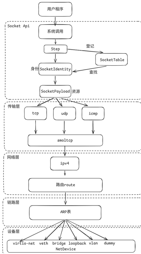
图 23 网络栈概述
